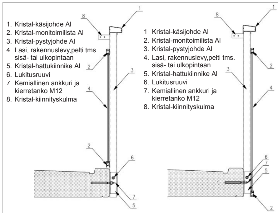
Kristal-kaide parvekelaatan etureunaan asennettuna
