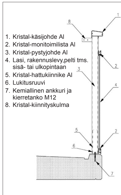
Kristal-kaide parvekelaatan päälle asennettuna
